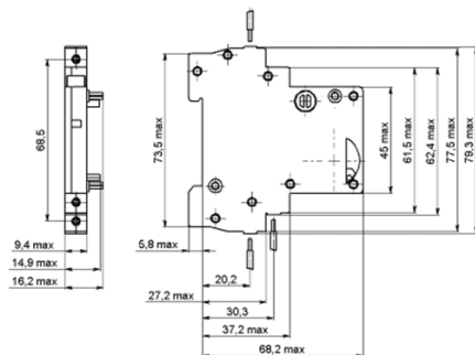
Рисунок 1 – Габаритные размеры МВК
