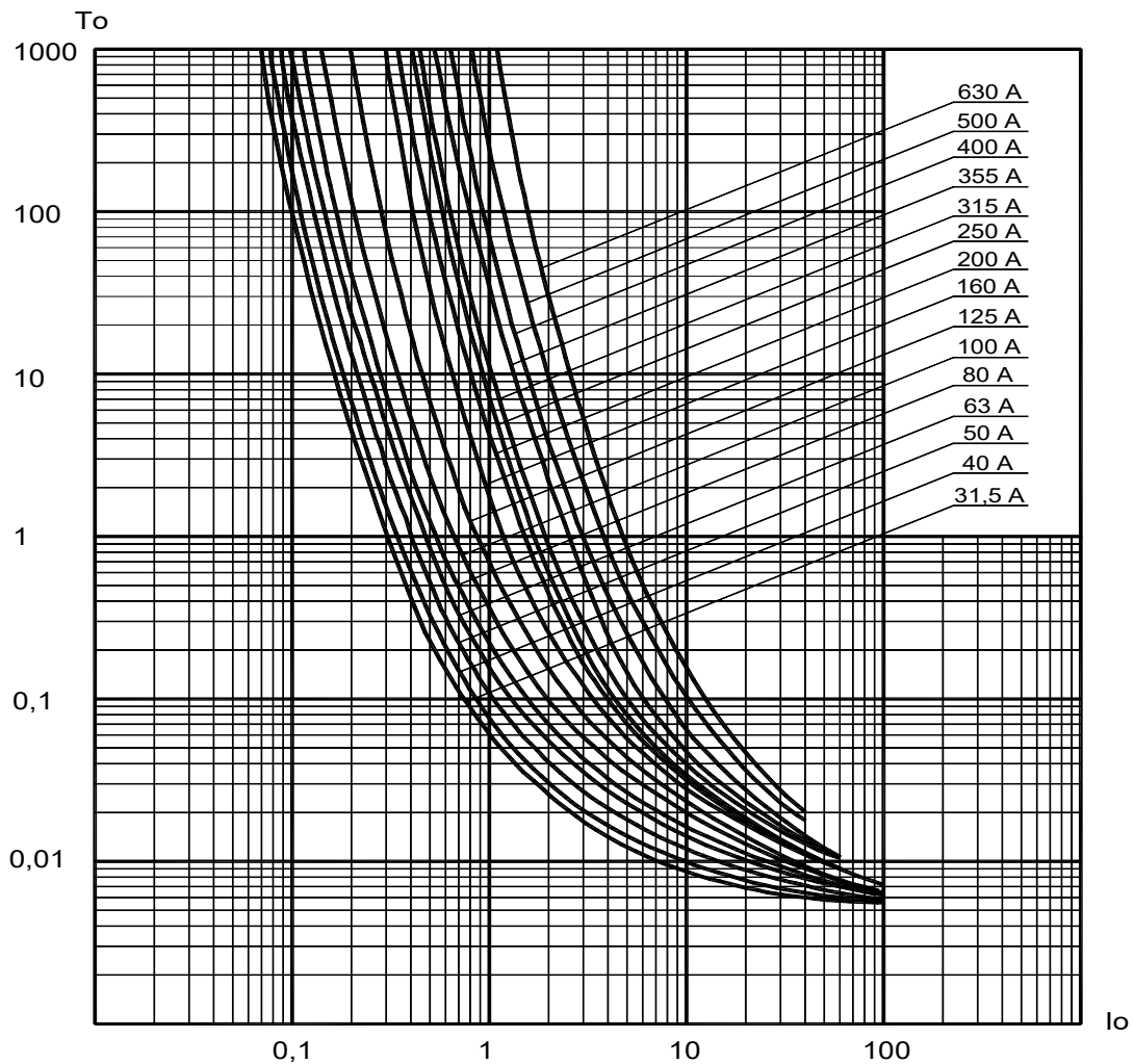
Рисунок Г.3 Предохранители типа ПН2-100, ПН2-250, ПН2-400 и ПН2-600.
